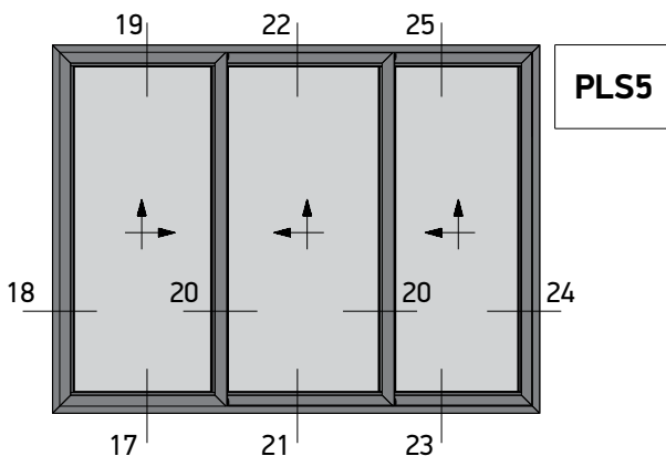
Three Sash Lift and Slide 45° Cut Right Τρίφυλλο Επάλληλο με κοπή 45° Δεξιά Ανάστρομενο
