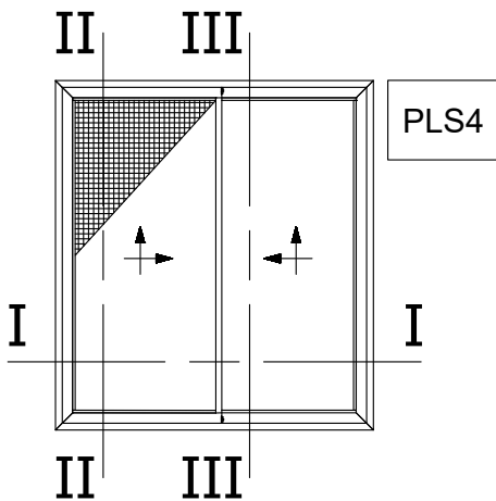
Two Sash Lift and Slide 90° Cut with Flyscreen Right Δίφυλλο Επτάλληλο με κοπή 90° και Σήτα Δεξιά Ανάσυρόμενο
