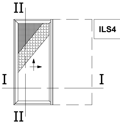
Single Sash Pocket Lift&Slide Window with Flyscreen and Shutter Μονόφυλλο Χωνευτό Ανασπώρομο με Σήτα και Παντζούρι
